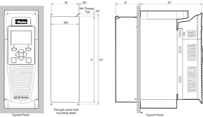
通孔安装
