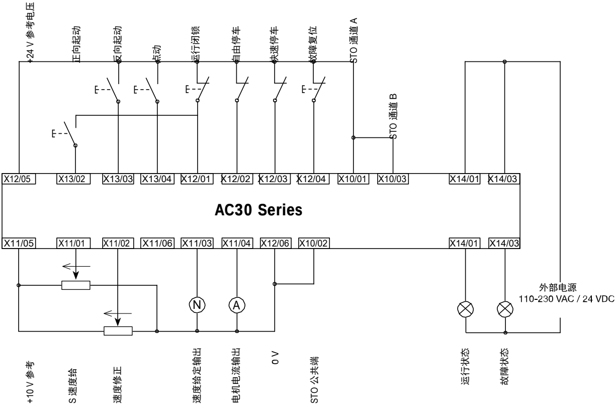
基本速度控制接线样例
