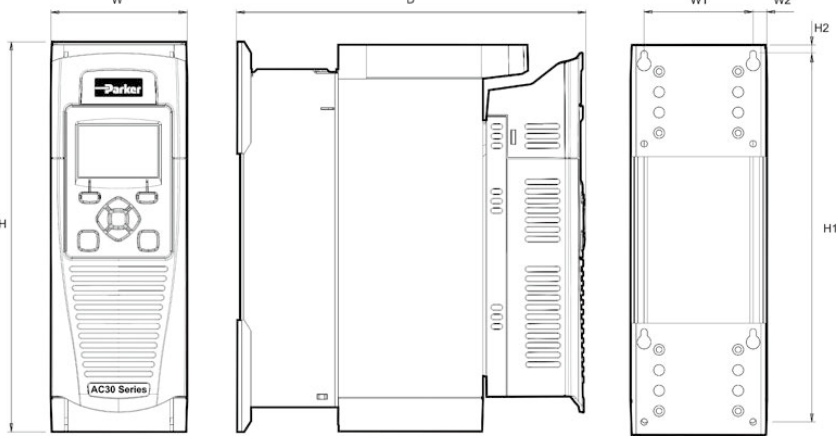
背板安装
