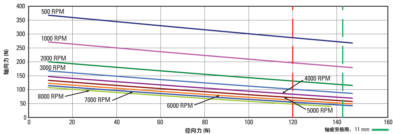
AKMH2 电机 20,000 小时 L10 轴承寿命
